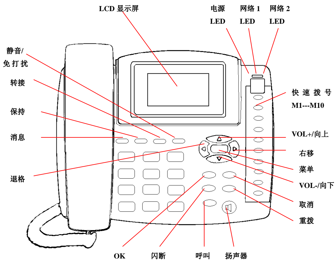
4.1.1 GP1266 话机面板示意图
