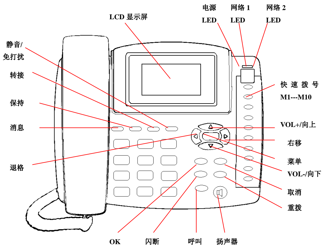
图 4.1.1 GP1266 话机面板示意图
